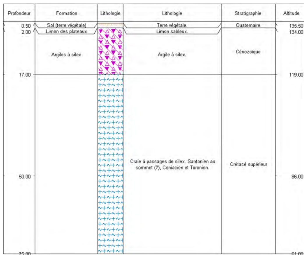
Figure 5. Sondage 00586X0020/F réalisé sur la commune de Pretot-Vicquemare
