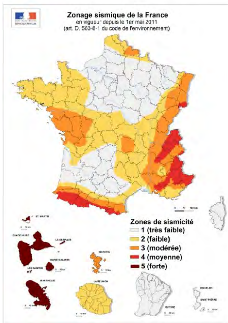
Figure 28. Zonage sismique de la France – source : BRGM
