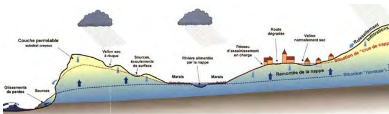
- Schéma d'une remontée de nappe - Source : SIGES Seine-Normandie
